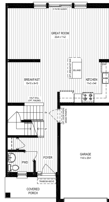
M1 - Main Floor
